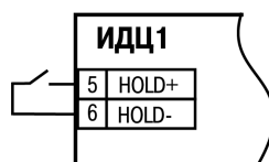
Рисунок 5.4 – Схема подключения коммутирующего устройства к прибору
