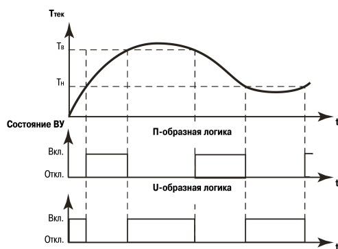
Рисунок 7.3 – Типы логики при работе ЛУ
