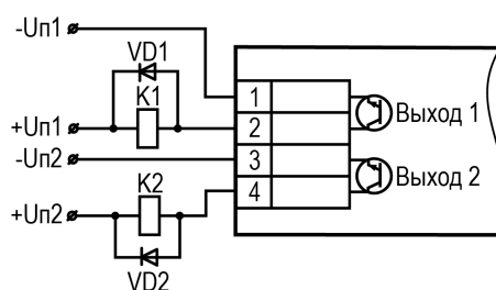
Рисунок 5.3 – Схема подключения реле к прибору
