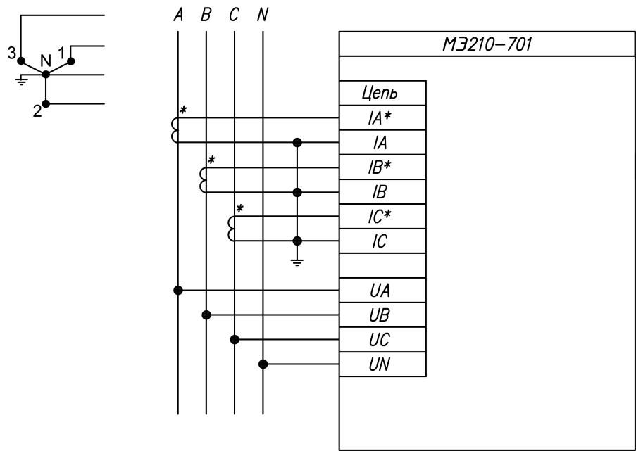
Рисунок 5.7 – Схема подключения 9S
