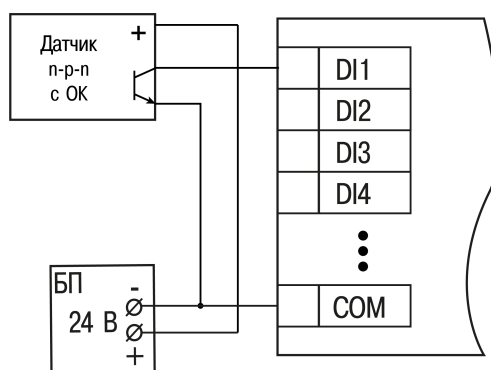
Рисунок 5.9 – Подключение транзисторов n-p-n
