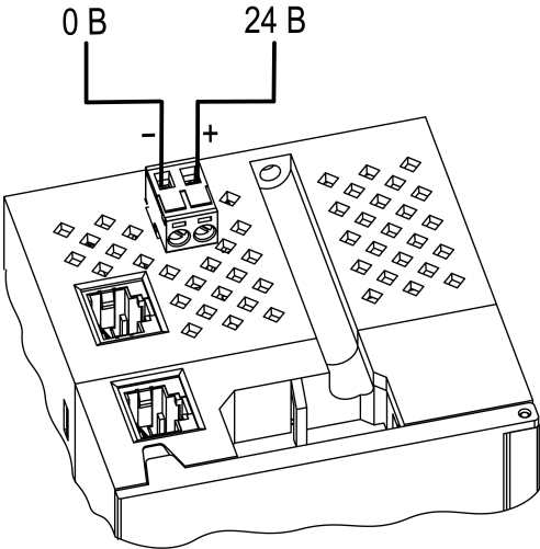
Рисунок 5.3 – Назначение контактов питания
