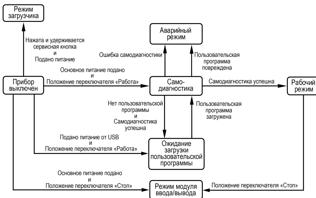
Рисунок 7.7 – Схема переходов между режимами работы
