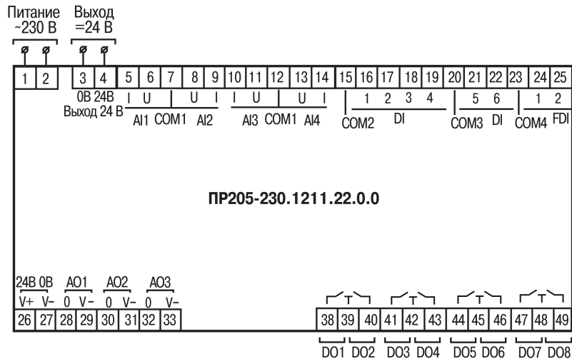
Рисунок А.5 – Расположение контактов для PR205-230.1211.22.0.0
