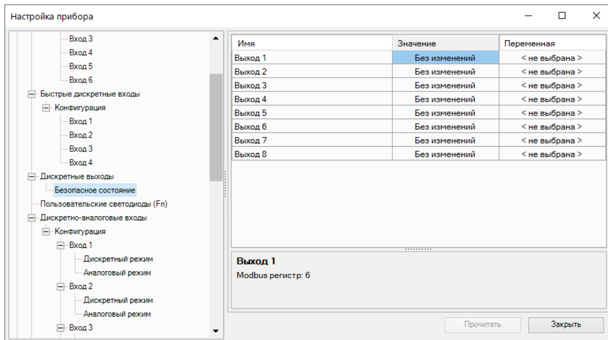
Рисунок 4.14 – Настройка безопасного состояния дискретных выходов
