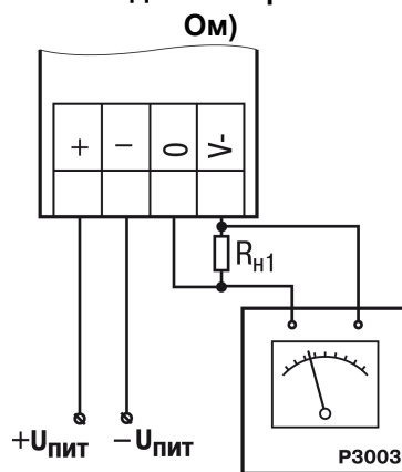
Рисунок В.4 – Схема подключения нагрузки к ВЭ для юстировки сигналов типа «0...10 В» ( R_n > 600 \text{ Ом} )
