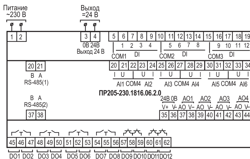
Рисунок А.12 – Расположение контактов для ПР205-230.1816.06.2.0
