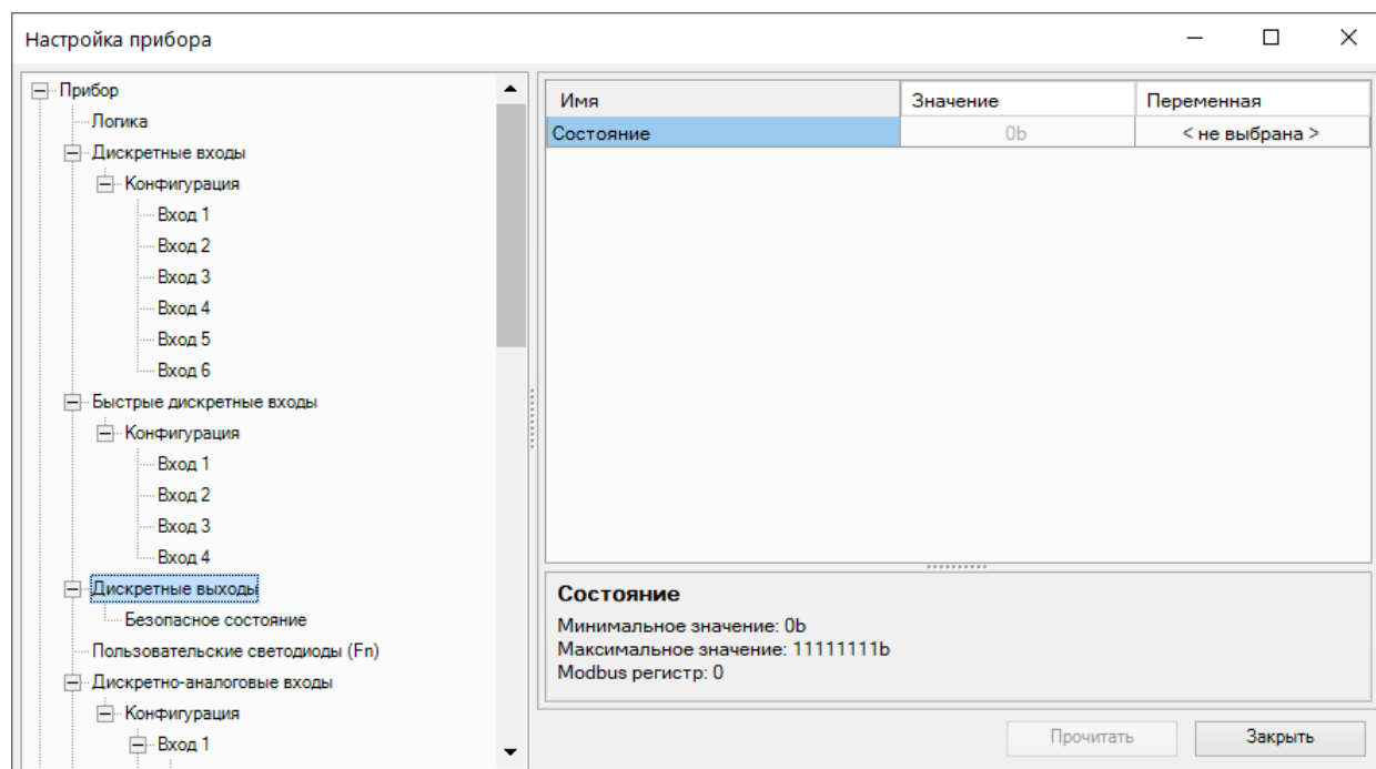
Рисунок 4.13 – Состояние дискретных выходов
