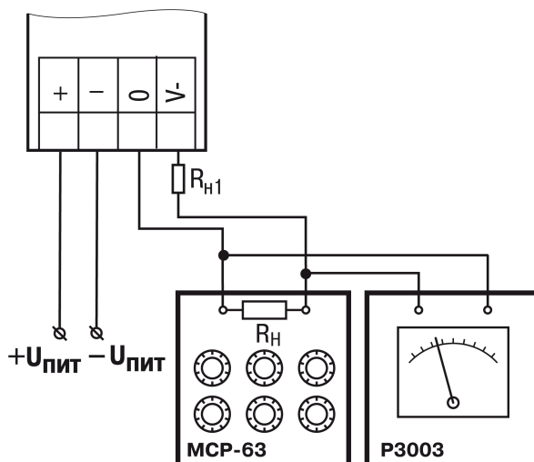
Рисунок В.3 – Схема подключения к ВЭ для юстировки сигналов типа «4...20 мА» ( R_n < 600
