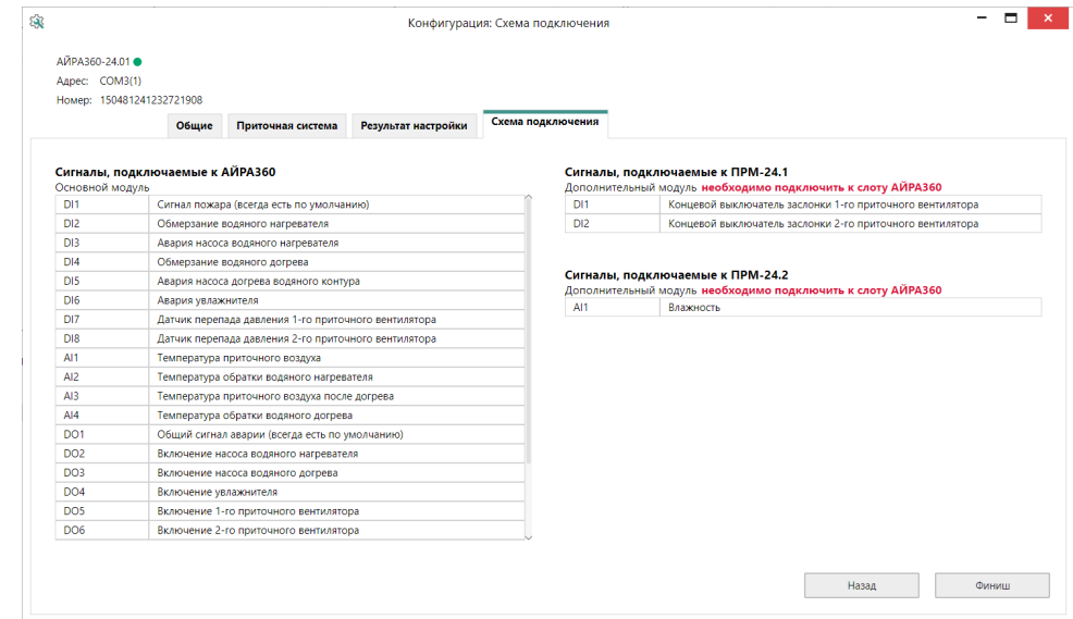
Рисунок 13.6 – Пояснения к схеме подключения
