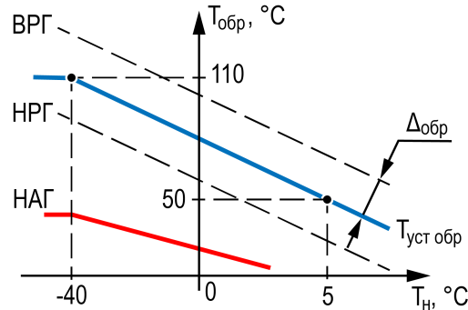
Рисунок 10.6 – График T_{обр}(T_n)
