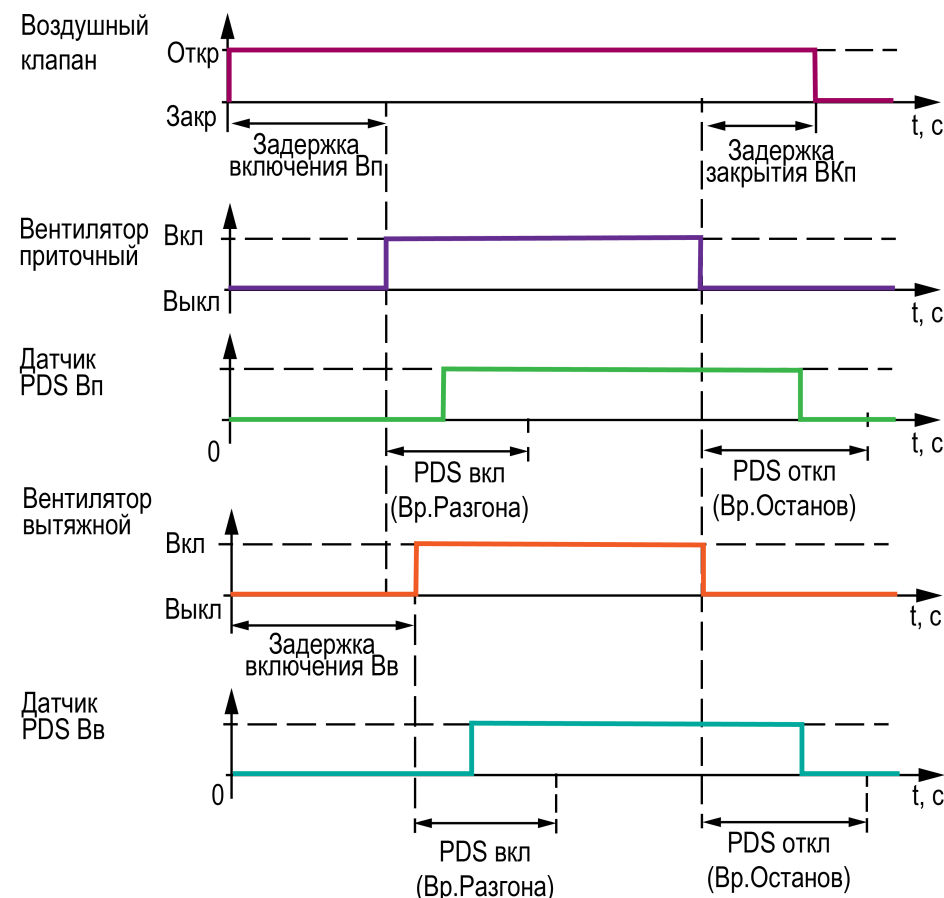
Рисунок 10.3 – Управление вентиляторами
