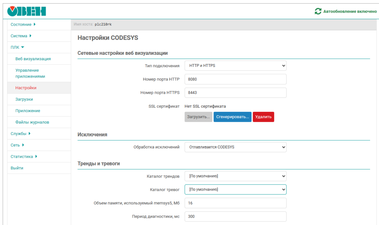
Рисунок 5.8 – Страница «Настройки»
