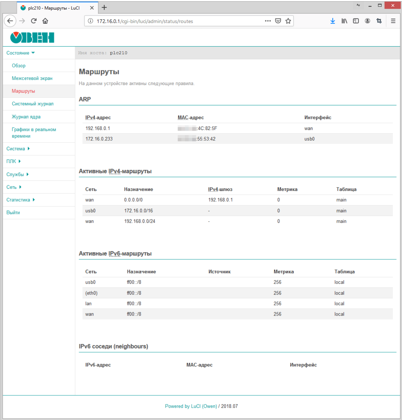
Рисунок 3.13 – Страница «Маршруты»
